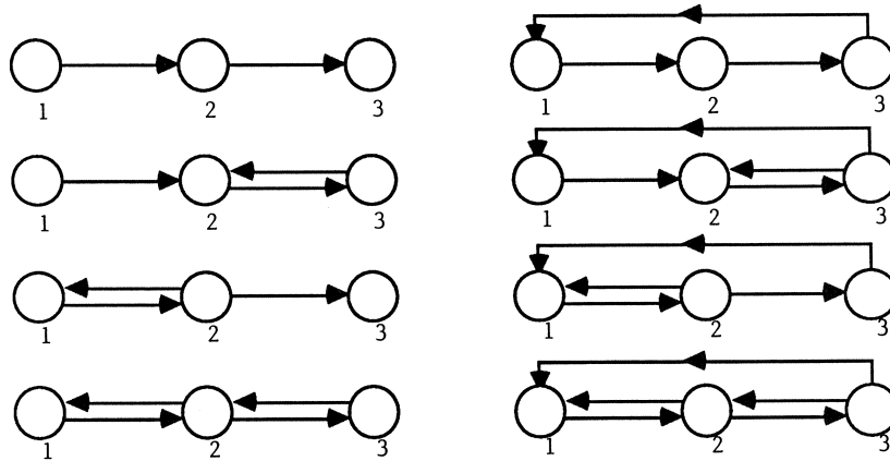
fig. 7.5.1. 8 possible choices for H in lemma 7.5.4.
